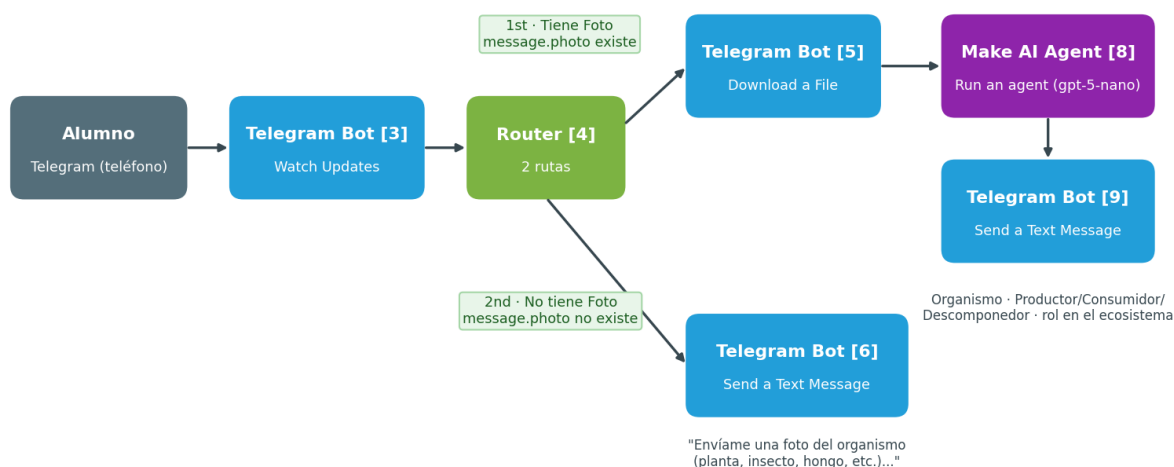
Figura 2. Diagrama de flujo del escenario y filtros del Router.
